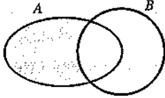
A \cap B Kümesi
