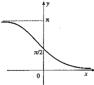
\operatorname{arccot} : \mathbb{R} \rightarrow [0, \pi) fonksiyonunun grafiği
