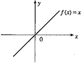
I_R fonksiyonunun grafiği
