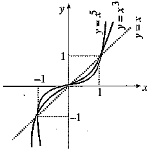
Bazı tek kuvvet fonksiyonlarının grafikleri
