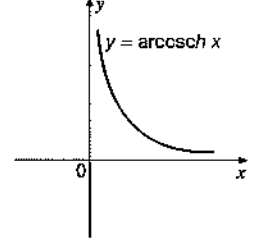
y = \operatorname{arccsch} x in grafiği
