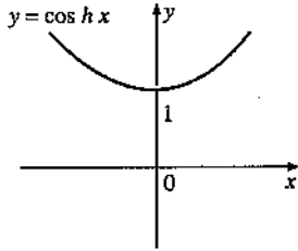
y = \cosh x in grafiği
