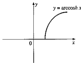
y = \operatorname{arccosh} x in grafiği
