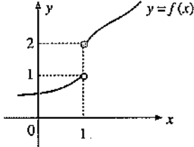
x = 1 de sıçrama süreksizliği
