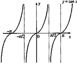
f(x) = \tan x in grafiği
