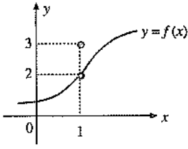
x = 1 de kaldırılabilir süreksizlik
