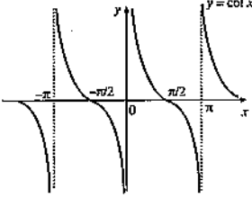
f(x) = \cot x in grafiği
