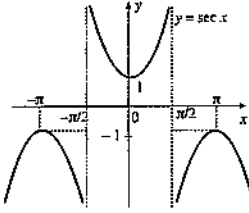
f(x) = \sec x in grafiği
