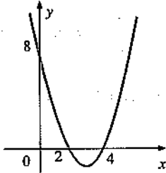
y = x^2 - 6x + 8 in grafiği
