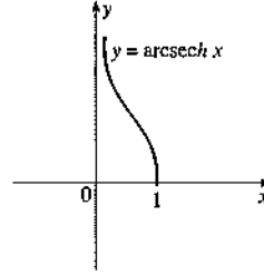
y = \operatorname{arcsech} x in grafiği
