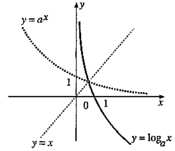
0 < a < 1 için y = \log_a x in grafiği
