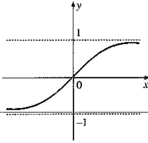
y = \tanh x in grafiği
