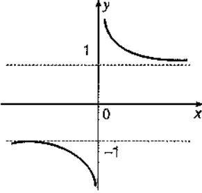
y = \coth x in grafiği
