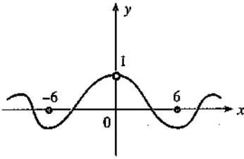
y = \frac{\sin x}{x} in grafiği
