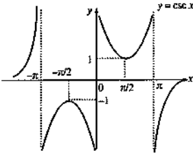
f(x) = \csc x in grafiği
