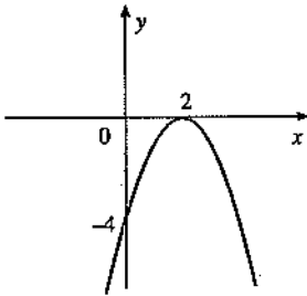
y = -x^2 + 4x - 4 in grafiği
