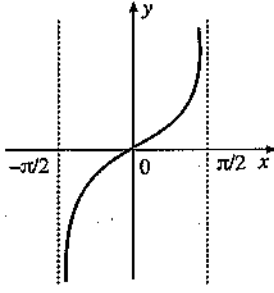
\tan : \left(-\frac{\pi}{2}, \frac{\pi}{2}\right) \rightarrow \mathbb{R} fonksiyonunun grafiği
