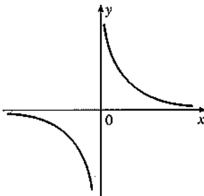
y = \operatorname{csch} x in grafiği
