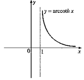
y = \operatorname{arccoth} x in grafiği
