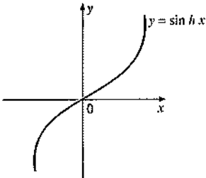
y = \sinh x in grafiği
