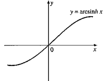
y = \operatorname{arsinh} x in grafiği
