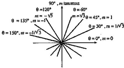
Çeşitli eğim açıları ve eğimler
