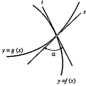
İki eğri arasındaki açı
