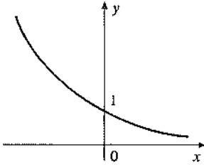
0 < a < 1 için y = a^x in grafiği
