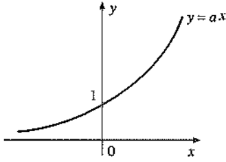
a > 1 için y = a^x in grafiği
