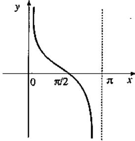
\cot : (0, \pi) \rightarrow \mathbb{R} fonksiyonunun grafiği
