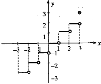
y = \lfloor x \rfloor in grafiği
