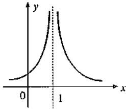
x = 1 de sonsuz süreksizliği
