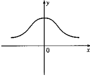
y = \operatorname{sech} x in grafiği
