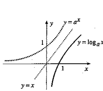
a > 1 için y = \log_a x in grafiği
