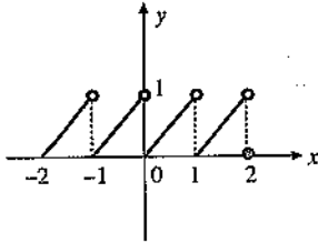
y = x - \lfloor x \rfloor in grafiği
