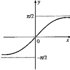
\arctan : \mathbb{R} \rightarrow \left(-\frac{\pi}{2}, \frac{\pi}{2}\right) fonksiyonunun grafiği
