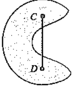
Konveks olmayan küme
