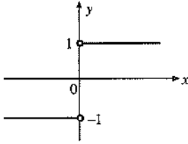
f(x) = \frac{x}{|x|} in grafiği
