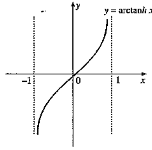
y = \operatorname{arctanh} x in grafiği
