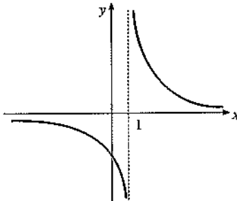
y = \frac{4}{x-1} fonksiyonunun grafiği
