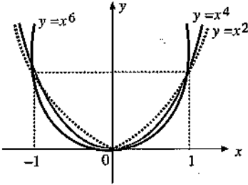
Bazı çift kuvvet fonksiyonlarının grafiği
