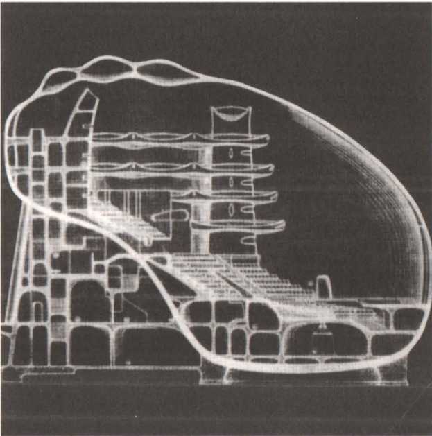
Evrensel Tiyatro, kesit, 1961.
