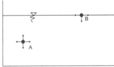
Şekil 2.14. Sıvı içerisindeki ve yüzeyindeki moleküllere etkili kuvvetler
