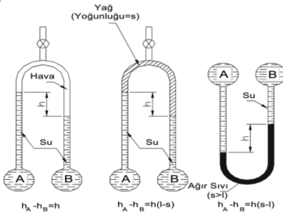
Diferansiyel manometreler
